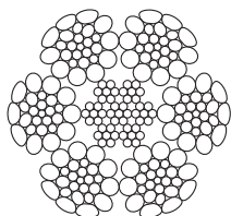
6x26KKWS+IWRC
