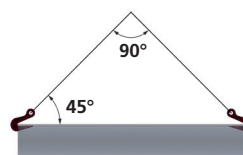
Fig.2** Portata max 2 ganci 10 t Max load 2 hooks 10 t
