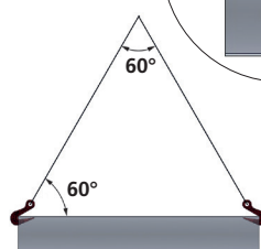
Fig.1* Portata max 2 ganci 2,8 t Max load 2 hooks 2.8 t
