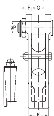
Con dado e coppiglia With bolt and split pin
