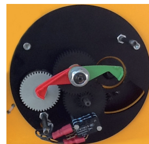
Fincorsa facilmente regolabile ed affidabile. Limit switch very easy to adjust and extremely reliable.
